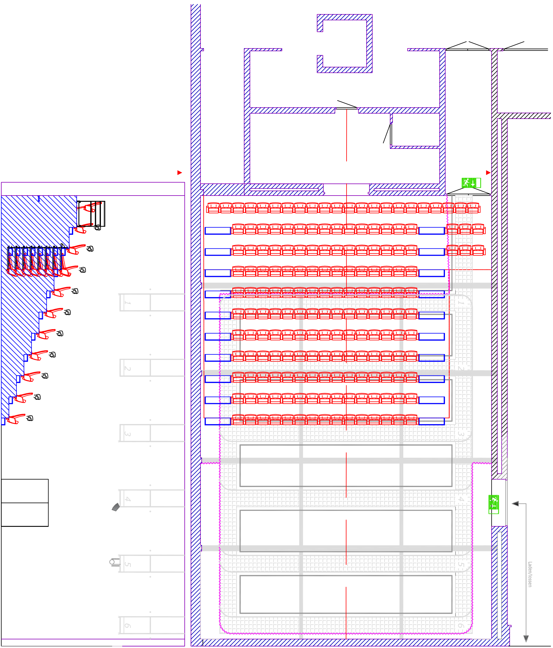
A3, 1:100, 360° Stadstheater Zoetermeer, Kleine Zaal
